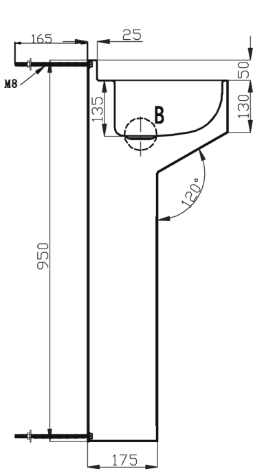
A-A
