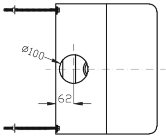
Вид снизу
